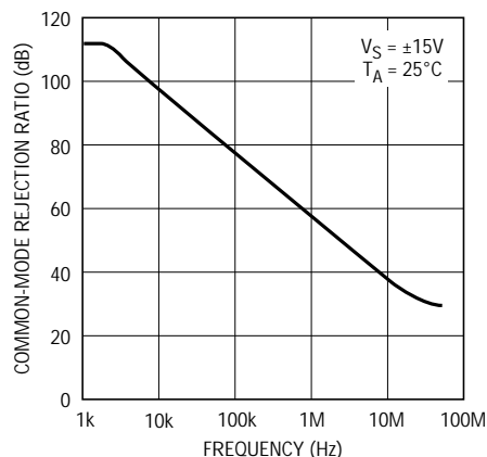
LT1221 • TPC10
