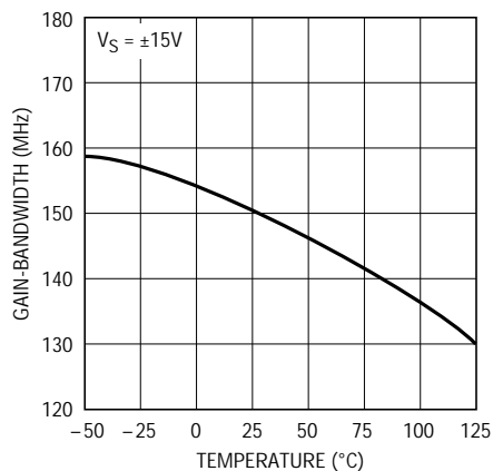
LT1221 • TPC16
