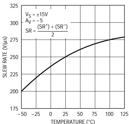
LT1221 • TPC19
