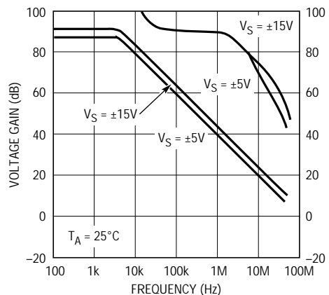
LT1221 • TPC13
